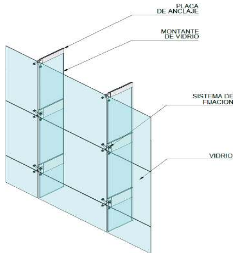
Figura 4. Sistema suspendido
